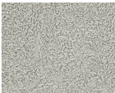
Helium
